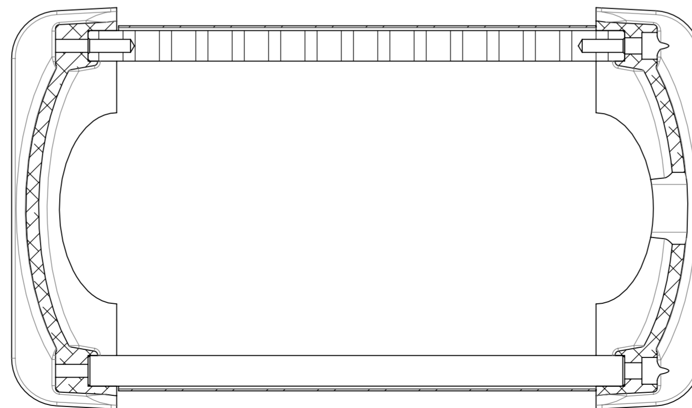
SEZIONE C-C
