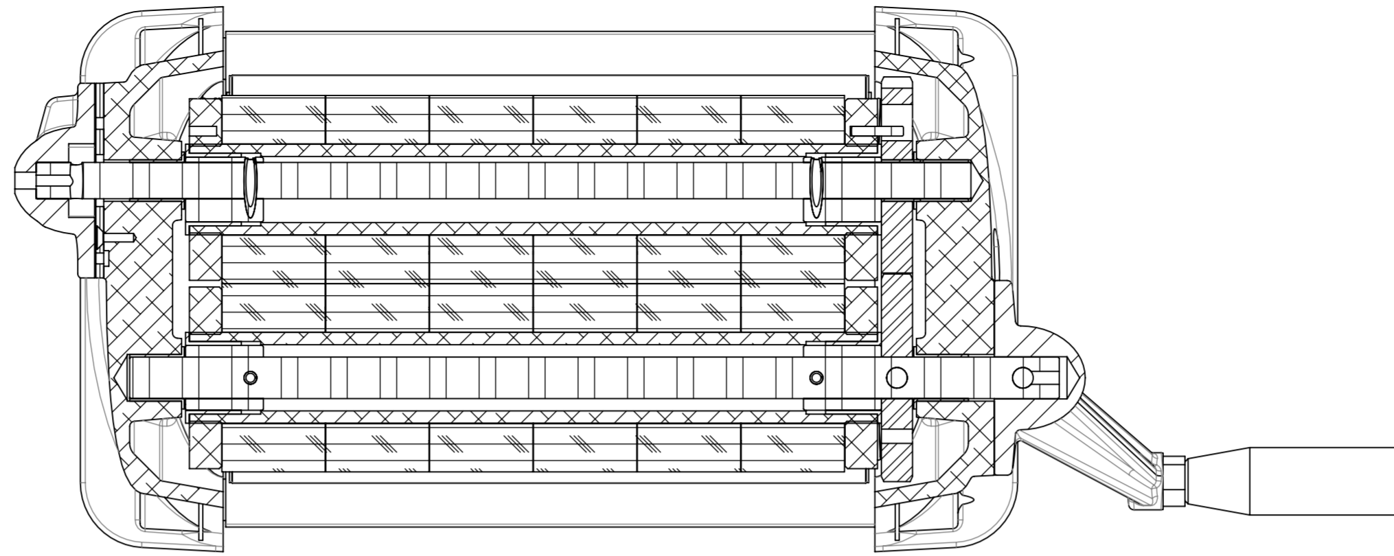
SEZIONE A-A
